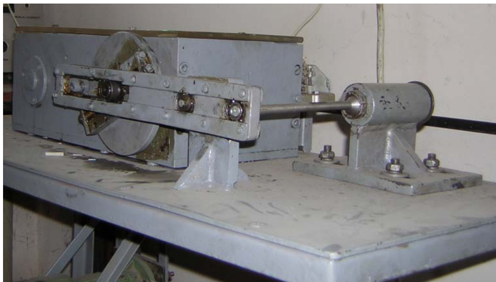
Masina de incercat la oboseala prin incovoiere plana
