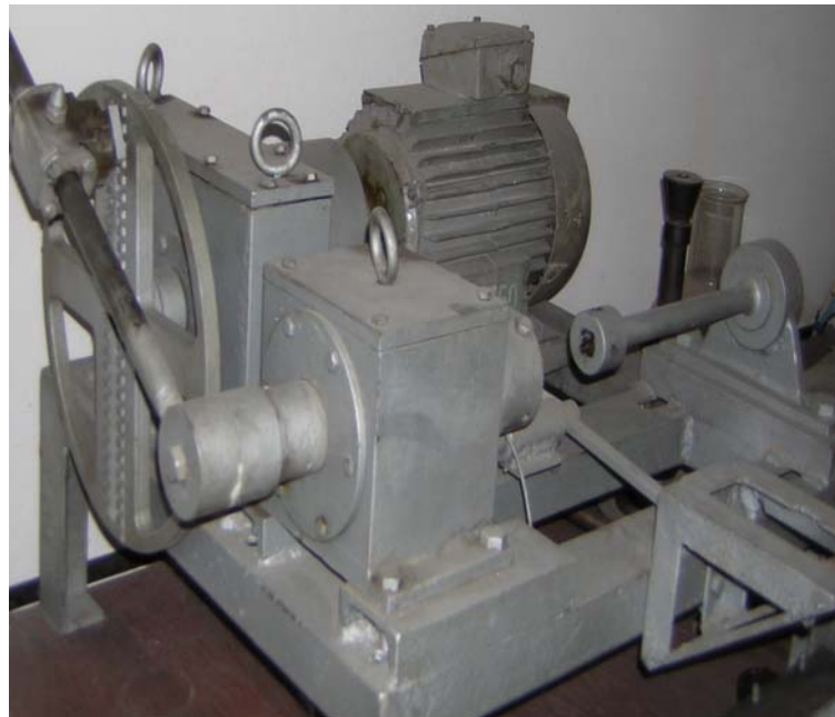
Masina de incercat la oboseala prin torsiune
